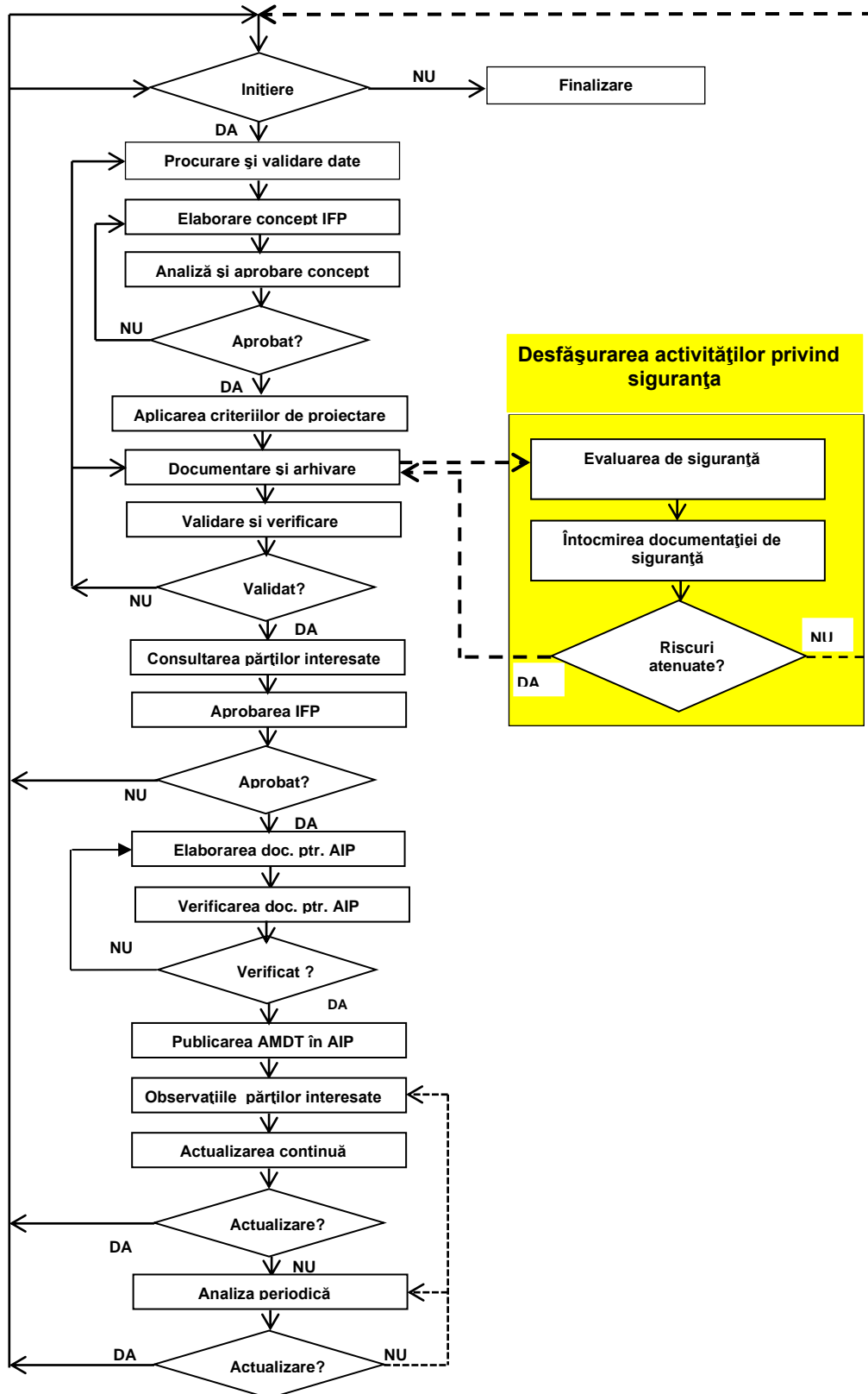
Figura 2. Schema logică a procesului IFP
